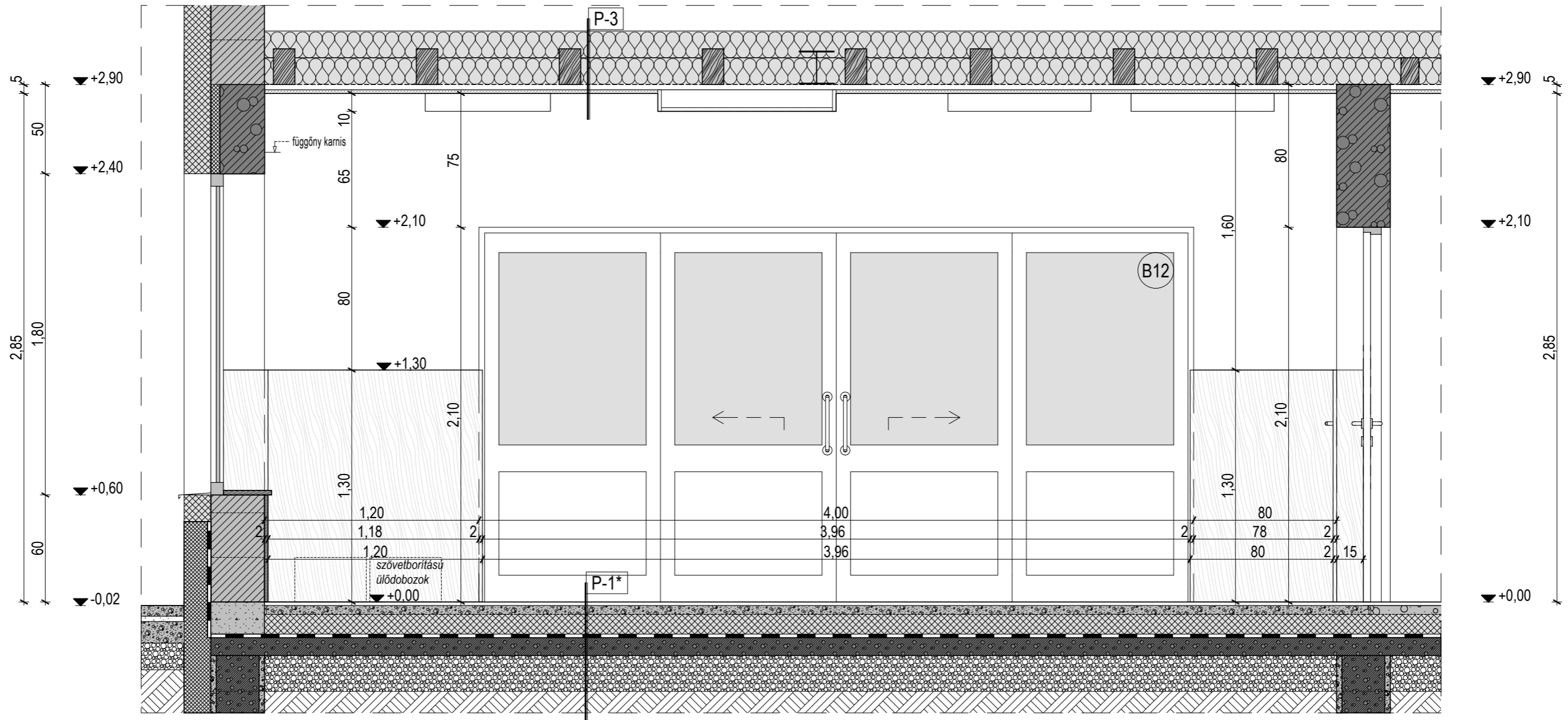
F - 1.6 FOGLALKOZTATÓ FALNÉZET M 1:25
