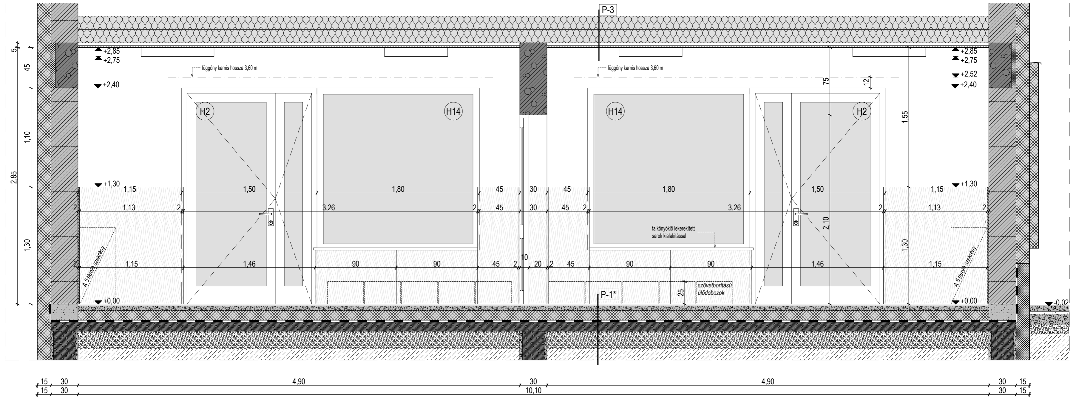
F - 1.3 FOGLALKOZTATÓ FALNÉZET M 1:25
