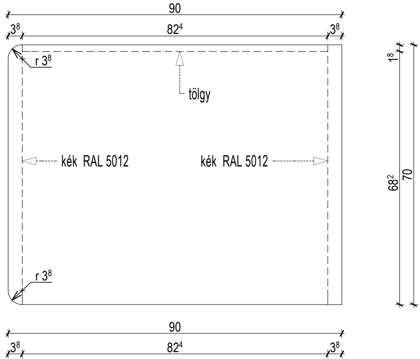
OLDALNÉZET M 1:10
