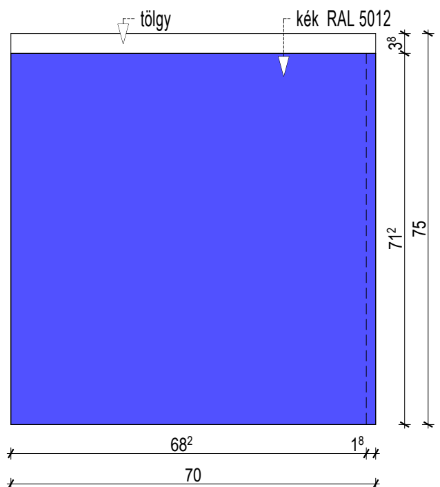
OLDALNÉZET M 1:10
