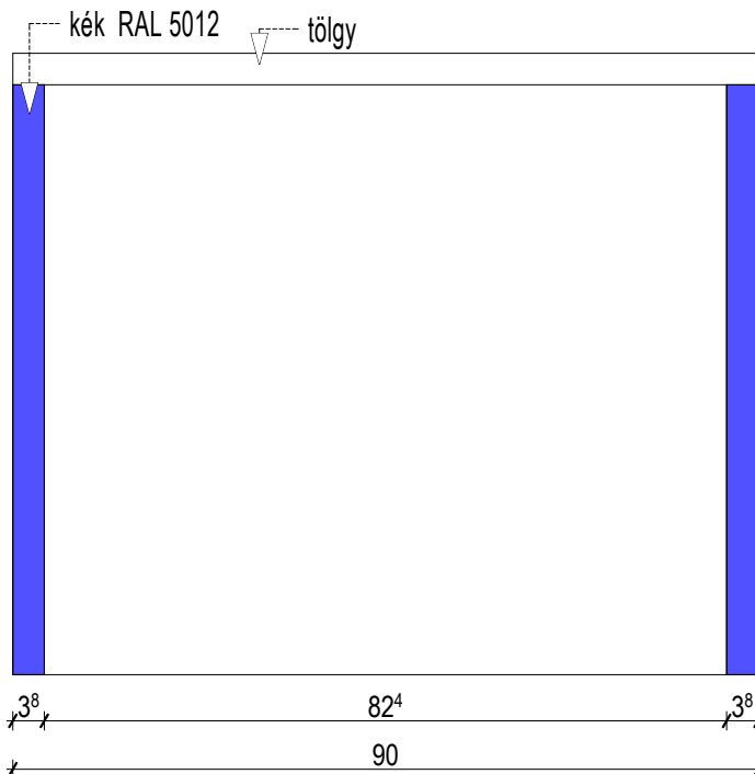
ELÖLNÉZET M 1:10
