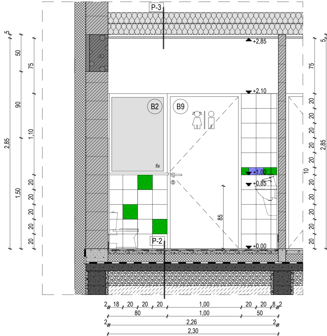
F - 3.4 GYEREK FÜRDŐ FALNÉZET M 1:25
