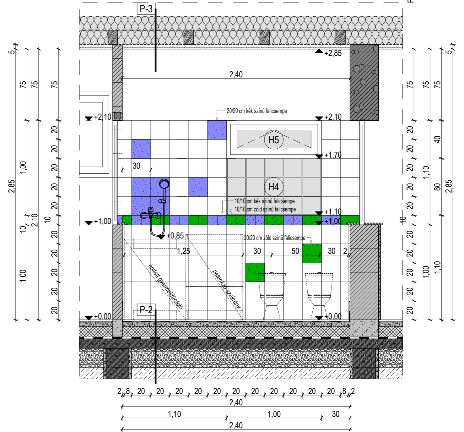
F3.3 GYEREK FÜRDŐ FALNÉZET M 1:25
