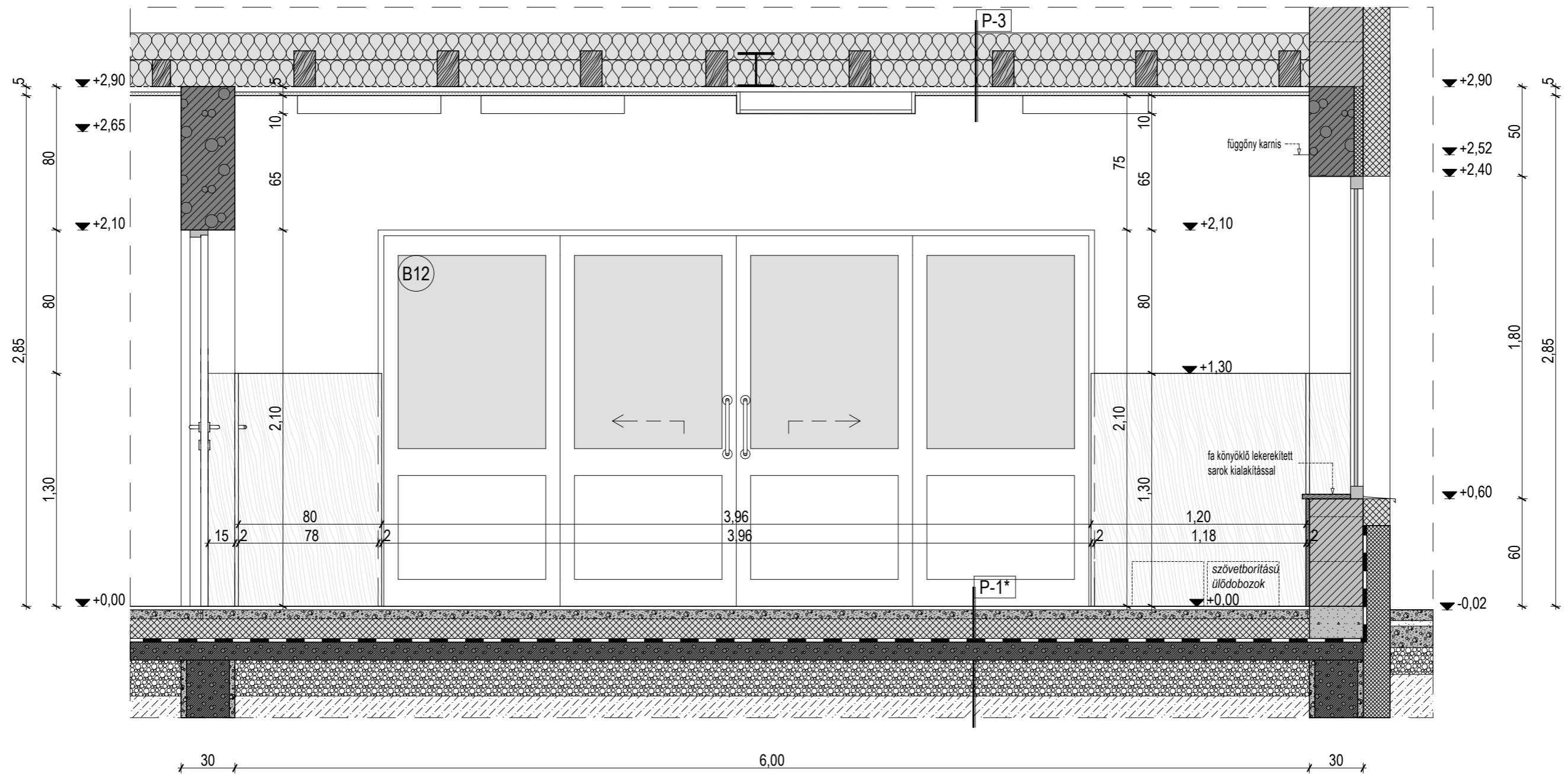
F - 1.2 FOGLALKOZTATÓ FALNÉZET M 1:25
