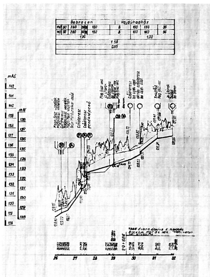
5. ábra: Kondoros csatorna hossz-szelvénye
