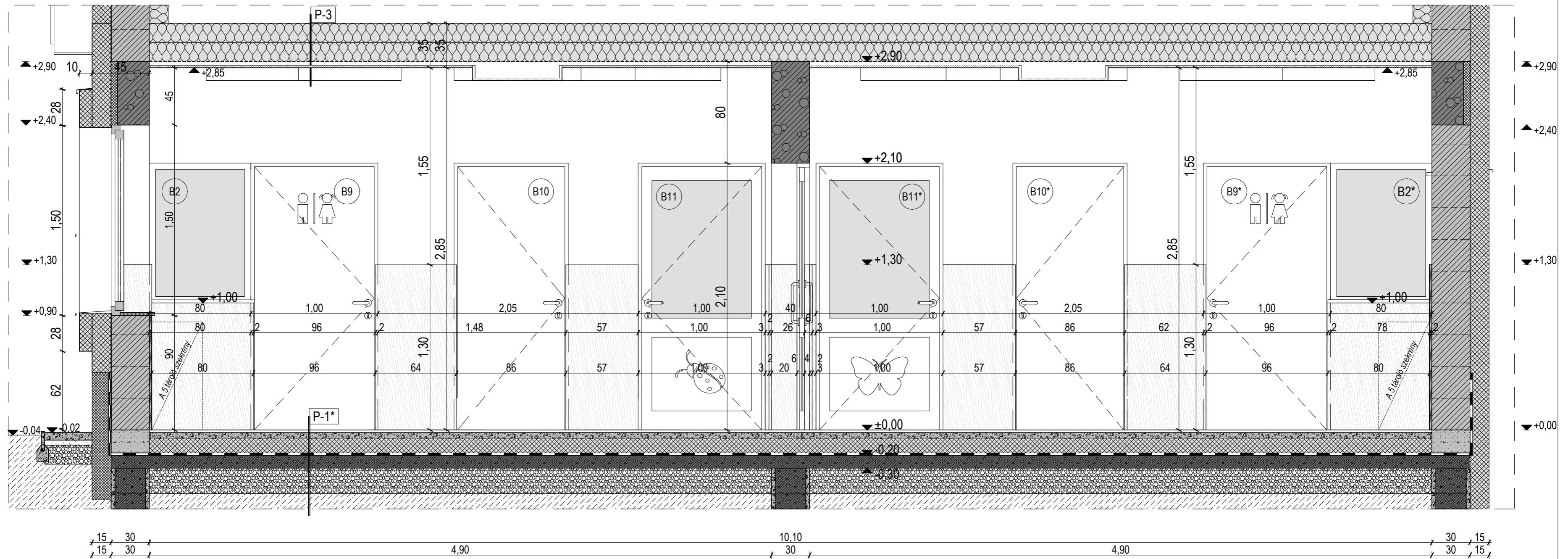
F - 1.5 FOGLALKOZTATÓ FALNÉZET M 1:25
