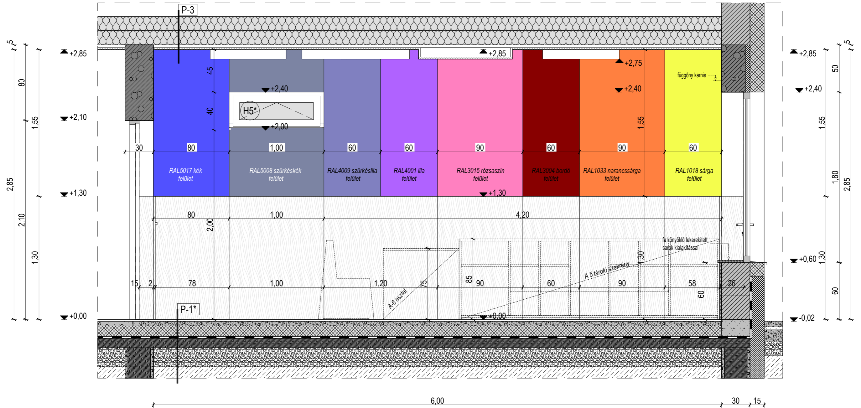
F - 1.4 FOGLALKOZTATÓ FALNÉZET M 1:25
