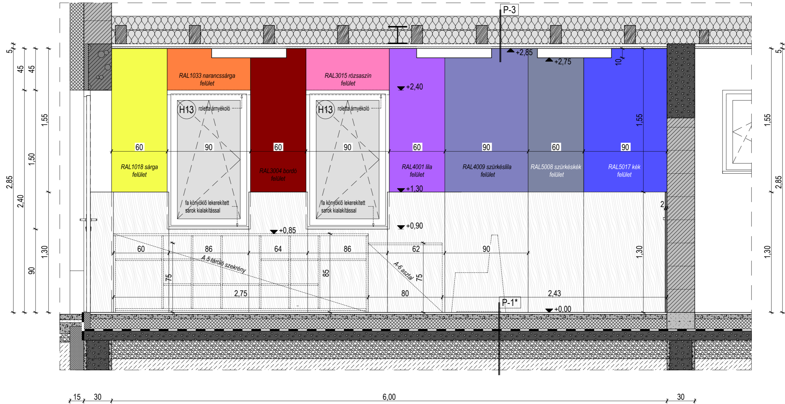
F - 1.1 FOGLALKOZTATÓ FALNÉZET M 1:25
